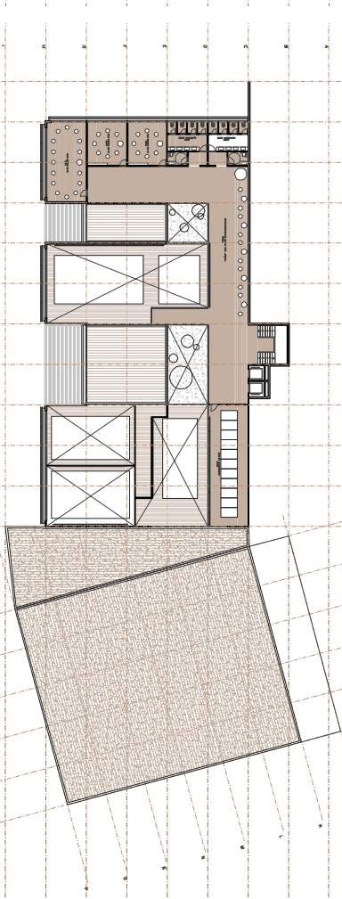
PLANTA CUARTA COTA +11,80m
