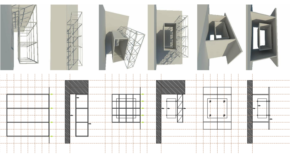
TIPOLOGÍA ESTRUCTURAL
