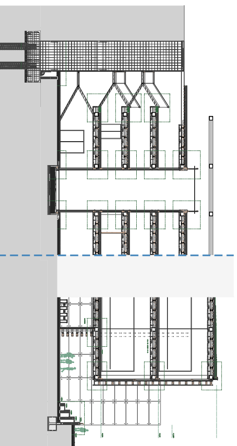
PLANTA TERCERA COTA +8.80m
