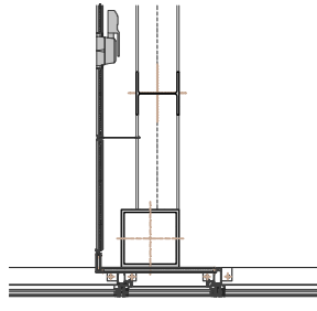
DETALLE V-12
