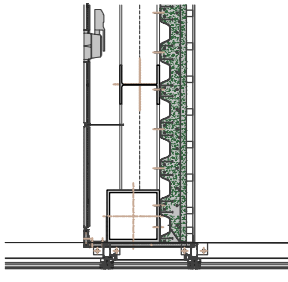
DETALLE V-11
