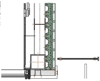
DETALLE V-11
