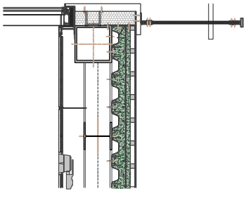
DETALLE V-18
